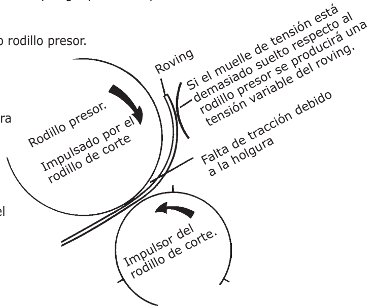
Disposición del Muelle del Rodillo Presor
