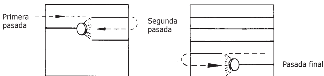
Ilustración esquemática mostrando el 50% de solapamiento en tiras y capas
