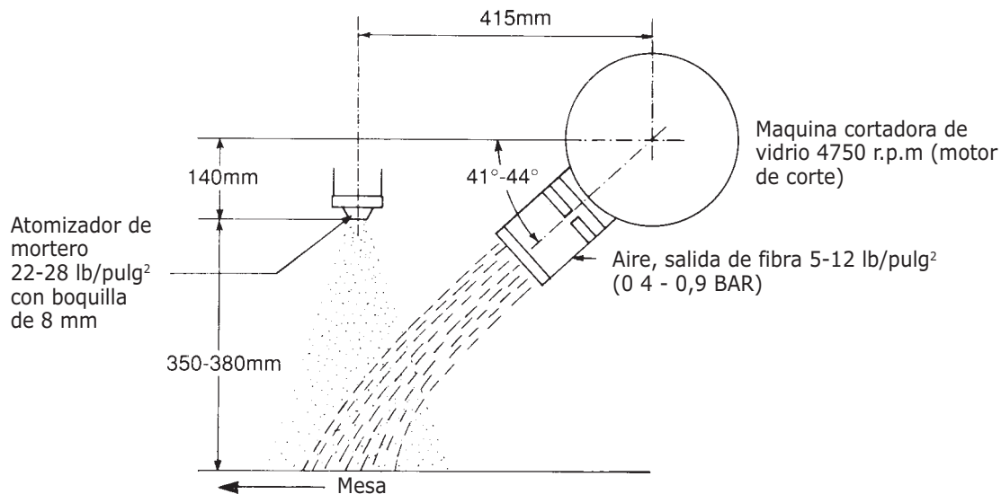
Disposición del Conjunto de Proyección con un único cortador
