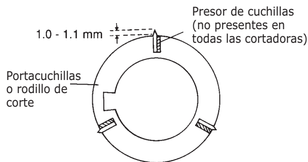
Disposición de las cuchillas
