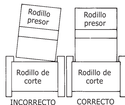
Disposición del rodillo presor
