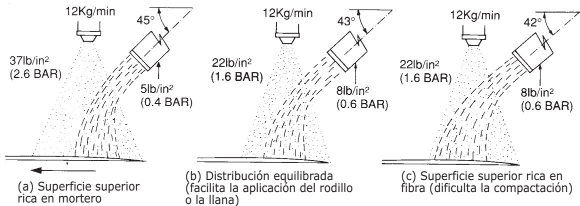
Ilustración del Efecto de Presión de Atomización y Ángulo de Deposición.
